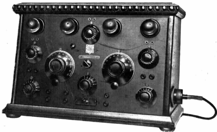
Ricevitore Neutrodina Rfe 10
