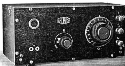
Radialba R 21 a due valvole
