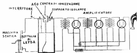
Diagramma del circuito
