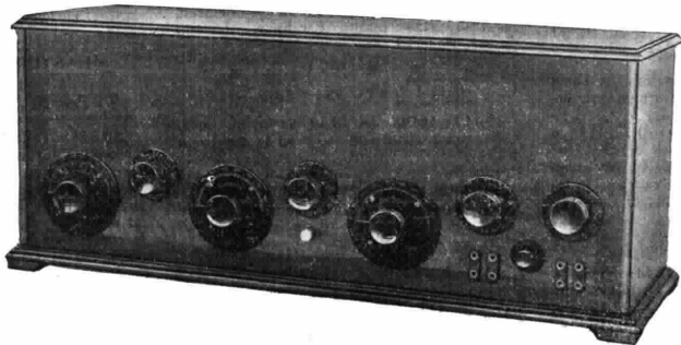
APPARECCHIO tipo R 14 per l'aereo con due stadi equilibrati di amplificazione in alta frequenza per la ricezione delle radio diffusiioni europee da metri 200 a 2000 in altoparlante anche durante il funzionamento di stazioni locali.
