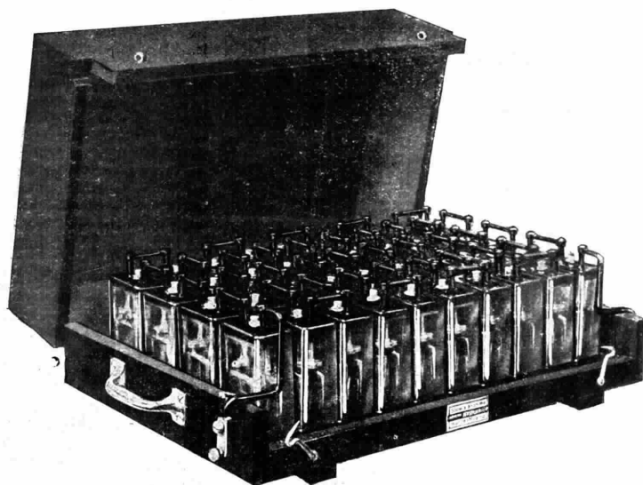
Batteria anodica d'accumul'atori - elementi in recipienti vetro - cassetta lucidata capacità 1,4 amperora - 80 volta.
