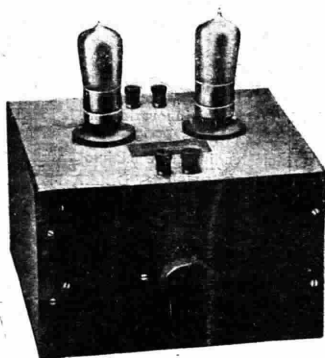
ALIMENTATORE di placca termoionico DEL VECCHIO Elimina la batteria anodica
