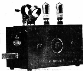
Ai apparecchio ricevente a 2 valvole
