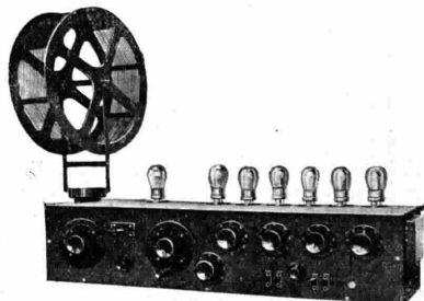
Il nuovissimo apparecchio a 7 valvole per la ricezione di stazioni lontane su quadro in altoparlante.
