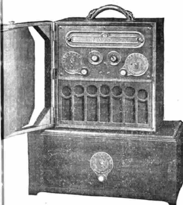
Apparecchio portatile Radiola 26
