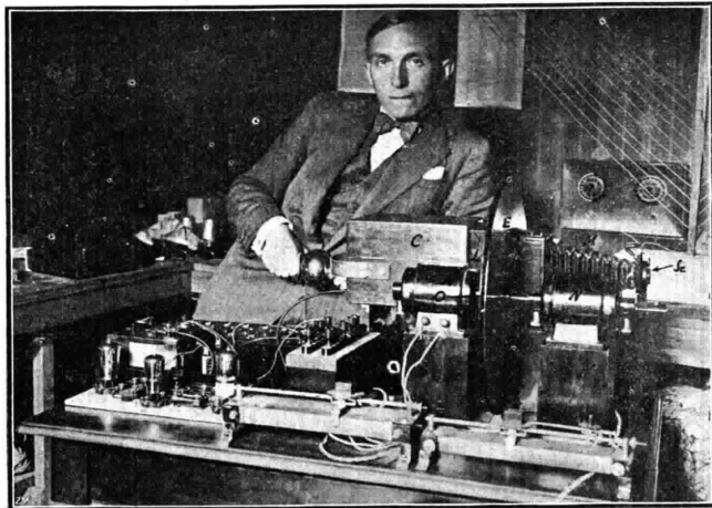
Apparecchiatura sperimentale di televisione Banfi M - macchina fotografica - E - disco esploratore - O - disco otturatore - L - sistema ottico C - cella fotoelettrica - N - motore elettrico
