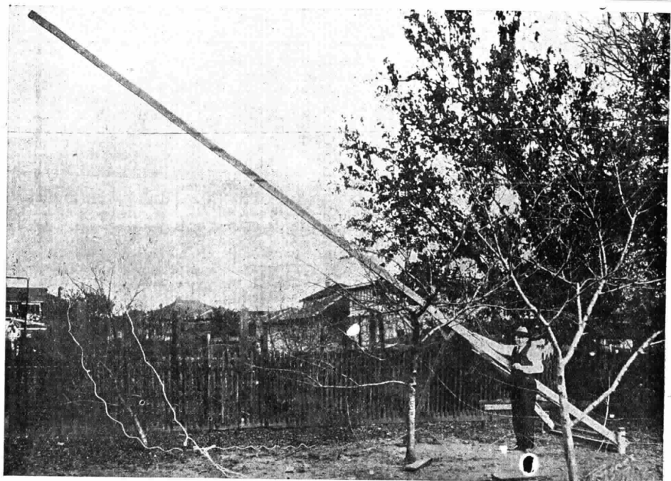
Questa antenna alta circa 10 metri è stata costruita dal sig. C. P. Gurgers, con pezzi di legname del diametro da 5-10 centimetri e della lunghezza di circa 4 metri. Alla base detti pezzi hanno la forma di Y. La base dell'antenna consiste in due robusti piccioli cacciati a forza nel terreno e distanti m. 1,50 l'uno dall'altro. Un ferro del diametro di 2,3 centimetri attraversa poi da banda a banda i piccioli e l'antenna, fungendo da perno, così che l'antenna può essere alzata e abbassata da una persona sola. Infine con solo pochi fili che servono da venti è ultimata una costruzione rigida e robustissima.
