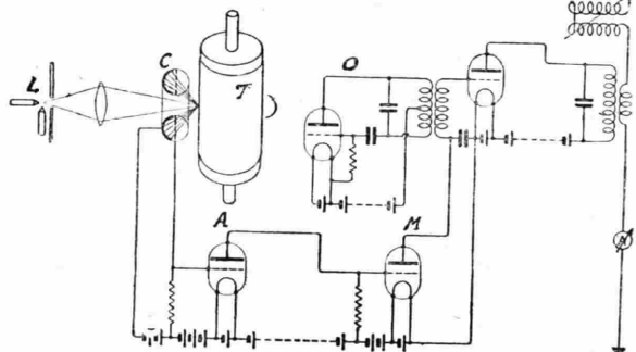
Fig. 1. — Dispositivo trasmettitore. L lampada ad arco — C cella fotoelettrica — T tamburo portante l'immagine originale — A amplificatore — M modulatore — O oscillatore pilota.
