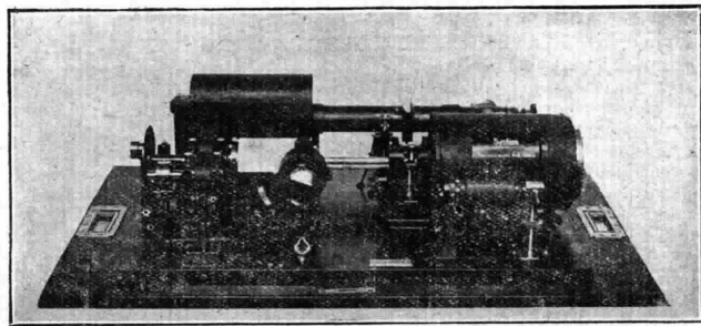
Fig. 6. — Parte principale complesso ricevente.
