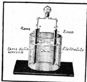
Fig. 7. — La pila elementare.
