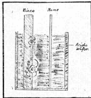
Fig. 9. — Impurità contenute negli elementi di una pila generano azioni locali che la esauriscono anche a circuito aperto.
