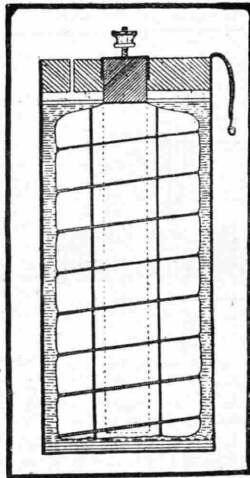
Fig. 8. — La pila a secco: il recipiente che costituisce l'elemento positivo o polo negativo.
