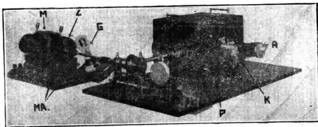
Fig. 5. — Complesso ricevente: M motore a corr. cont. — Z ruota a denti La Cour — MA bobine di comando sincronismo — G lampada al neon — P Nicol polarizzatore (interno al tubo) — K cella Karolus — A Nicol analizzatore e prisma a riflessione totale.
