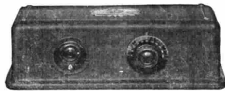
APPARECCHIO modello 35 - Tutto in metallo — Comporta un circuito a 6 valvole delle quali 3 amplificatrici in A.F. accordate-compensate - una detettrice - 2 amplificatrici in B.F. - un solo reostato per l'accensione delle valvole - UN SOLO COMANDO per la ricerca delle stazioni. Dimensioni cm. 41x15x16,50 - Peso Kg. 5,600.
