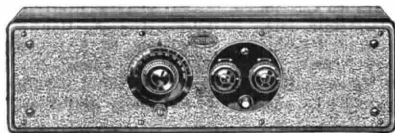
APPARECCHIO modello 30 — Comporta un circuito a 6 valvole delle quali 3 amplificatrici in A.F. accordate-compensate, una detettrice, due amplificatrici in B.F. - un reostato per l'accensione delle valvole A.F. - un reostato per l'accensione della valvola detettrice - UN SOLO COMANDO per la ricerca delle stazioni. Dimensioni cm. 49x15,50x15,50 - Peso Kg. 6 - Elegante cassetta palisandro luc.
