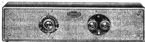
APPARECCHIO modello 32 - Portentoso — È veramente il migliore prodotto del mercato mondiale. Comporta un circuito a 7 valvole delle quali 4 amplificatrici in A.F. - una detettrice - 2 amplificatrici B.F. - un reostato per l'accensione delle valvole A.F. - un reostato per l'accensione della valvola detettrice - UN SOLO COMANDO per la ricerca delle stazioni. Dimensioni cm. 58x16x16,30 - Peso Kg. 7 - Elegante cassetta in palisandro luc.
