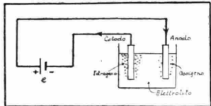
Fig. 9. — Il fenomeno dell'elettrolisi: la corrente elettrica decompone l'acqua nei suoi elementi costitutivi.
