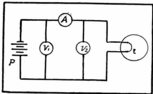
Fig. 29. - Inserzione di un voltmetro ed un amperometro in un circuito elettrico.
