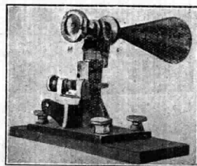
Fig. 3 - Montaggio dello specchio oscillante M al posto trasmettente.
