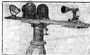
Fig. 2 Posto trasmettente disposto per impiegare la luce solare.
