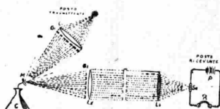
Fig. 1 - Schema della telefonia luminosa del Prof. Rankine
