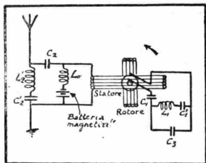
Fig. 49. — Costituzione schematica di un alternatore ad alta frequenza tipo Goldschmidt.
