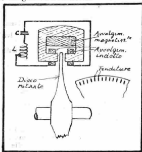
Fig. 48. — Costituzione schematica di un alternatore ad alta frequenza tipo Alexanderson.
