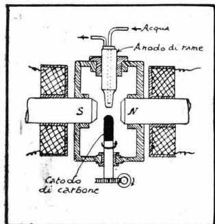
Fig. 54. — Costituzione pratica di un generatore ad arco.
