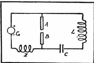
Fig. 52. — Circuito schematico di un generatore ad arco.
