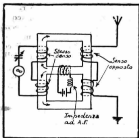
Fig. 50. — Costituzione schematica di un duplicatore di frequenza.
