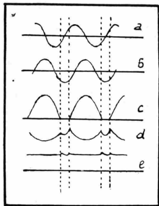
Fig. 55. — Diagramma di funzionamento del generatore ad arco.
