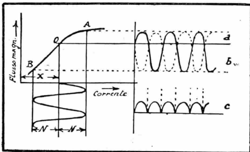
Fig. 51. — Diagramma di funzionamento di un duplicatore di frequenza.
