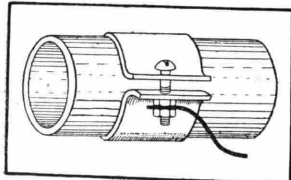
Fig. 80. - Presa di terra alla tubazione d'acqua potabile.
