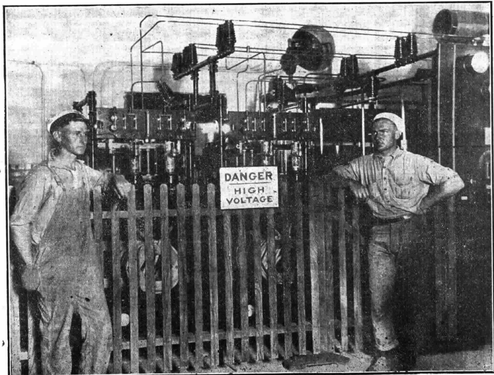
Complesso di quattro valvole trasmettenti da 20 Kw ciascuna, che hanno sostituito un generatore ad arco da 200 Kw
