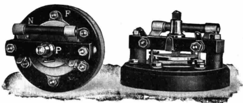
Equilibratore "SITI,,
