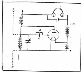
Fig. 99. — Triodo rivelatore montato in autodina (rigenerazione).
