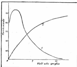
Fig. 123. - Paragone fra il rendimento dei due sistemi principali di rivelazione: 1 rettificazione di griglia; 2 rettificazione anodica.
