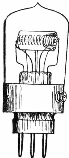
Valvola bigriglia di potenza DV 8 P impiegata nel circuito (2) per un dispositivo trasmettente ricevente duplex per radiotelegrafia. In questo circuito viene impiegato un tetrodo come oscillatore e ricevitore ed un triodo quale modulatore ed amplificatore.
