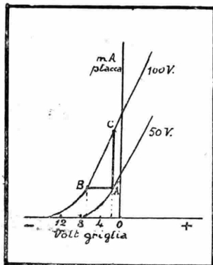
Fig. 120. - Diagramma dimostrativo del coefficiente d'amplificazione.
