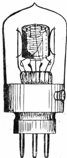
Valvola con catodo alimentata da corrente alternata "Volta 3,, impiegata nel circuito N. 1
