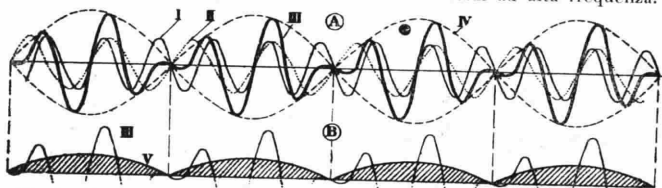
Fig. 5. - Rappresentazione grafica del fenomeno dei battimenti.
