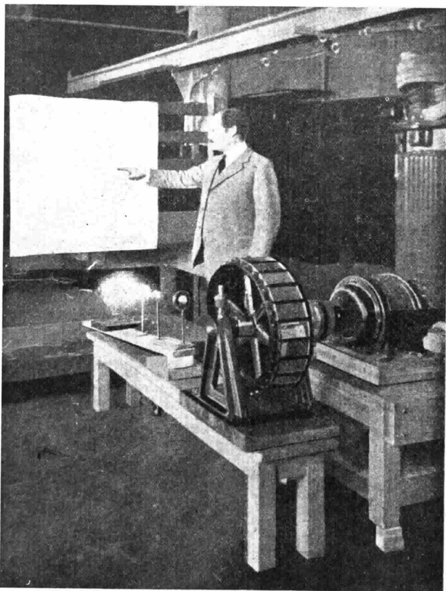
L'ing. Alexanderson con l'apparecchio di sua invenzione per radiotrasmettere le pellicole cinematografiche
