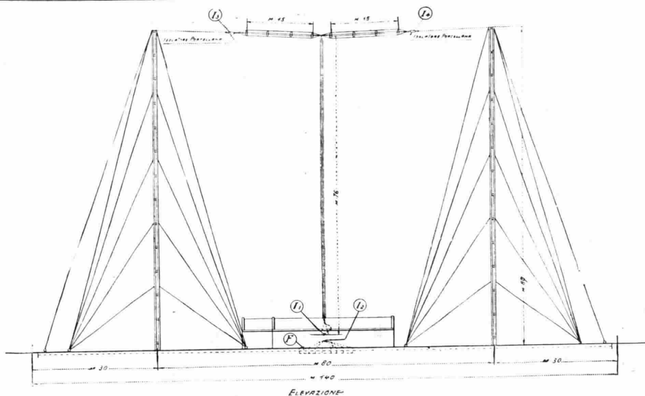
STAZIONE RADIOTELEFONICA di MILANO (Vigentino) - KW. 7 ANTENNA -
