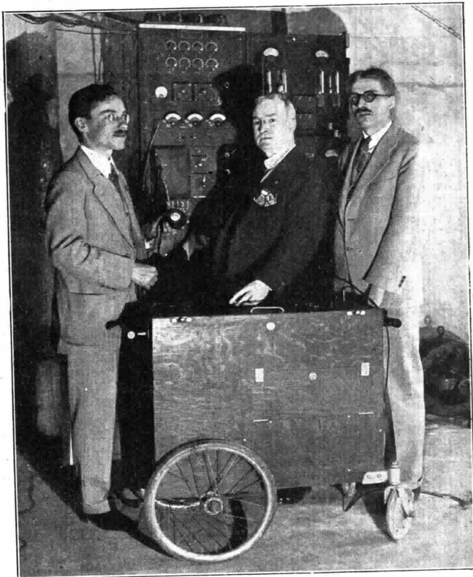
CON L'AUSILIO DI UN MICROFONO APPOGGIATO PRESSO IL CUORE DI UN PAZIENTE, È STATO POSSIBILE AMPLIFICARE CENTO MILIONI DI VOLTE IL SOFFIO CARDIACO, E FARLO COSÌ UDIRE AD UN'ADUNANZA DI MIGLIAIA DI PERSONE. LA NOSTRA FOTOGRAFIA MOSTRA IL COMPLESSO DEGLI AMPLIFICATORI E IL MICROFONO USATI IN TALE ESPERIMENTO.
