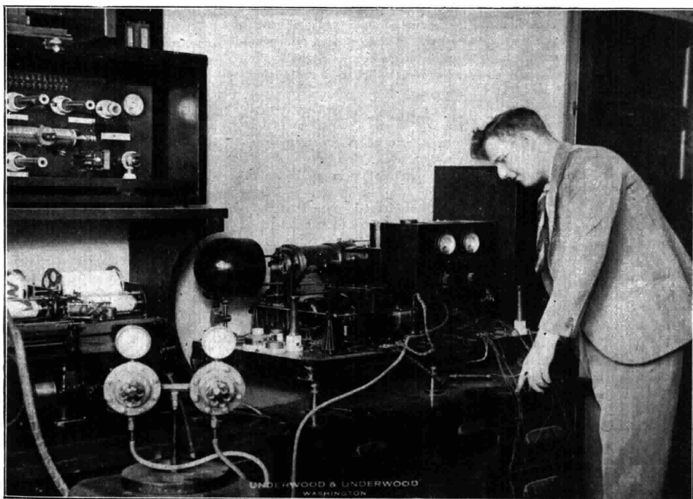
Negli Stati Uniti d'America il servizio di trasmissioni fototelegrafiche è ormai entrato in una fase di applicazione corrente. Ecco uno dei dispositivi normalmente usati per tali trasmissioni.
