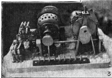
1) Complesso degli indicatori di inclinazione trasversale e longitudinale con relativo servomotore - 2) Organo stabilizzatore di quota - 3) Servomotore per la regolazione del motore ad essenza
