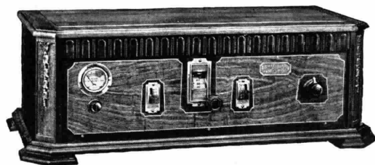
(6 Valvole UX 201 A - 2 Valvole UX 171 - 1 Valvola UX 280) VALVOLE NORMALI
