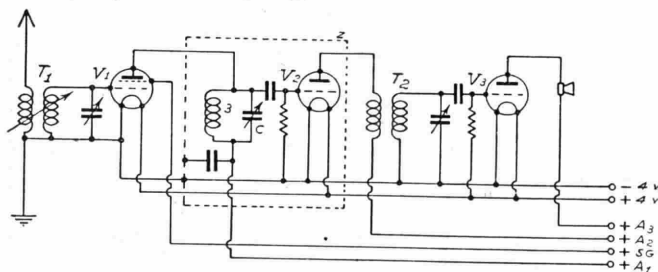
Fig. 1. — Circuito con due stadi ad A.F. di cui uno con valvola schermata. T e T_2 = trasformatori ad A.F.; 3 = bobina a nido d'api; V_1 = valvole schermate; V_2 e V_3 = triodi normali.
