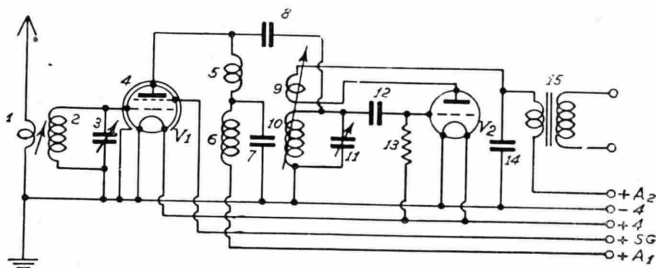
Fig. 2. — Circuito con uno stadio adB.F.; V_1 = valvola a placca schermata; 1-2 = variometro d'aereo; 5-6 = bobine di « choke »; 9 = bobina di reazione; 10 = bobina a nido d'api; 15 = trasformatore a B.F.; V_2 = triodo normale.
