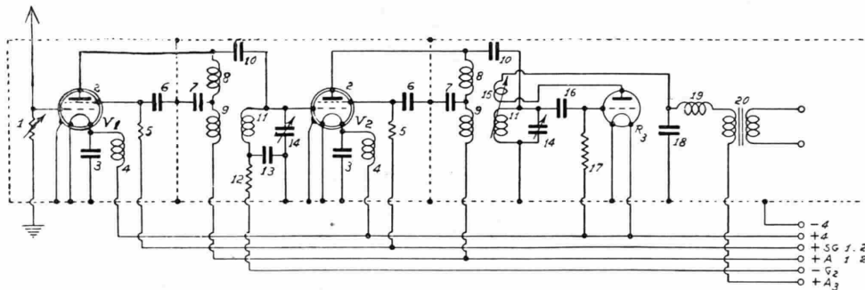
Fig. 4. — Circuito con due stadi ad A.F. a valvole a placca schermata. 1=resistenza variabile da 50.000 ohm; 4=choke di filo (60 spire filo 0,4 mm. diam. su mandrino 10 mm. diam. e 20 mm. lunghezza); 5 = resistenza 50.000 ohm; 8-9 = bobine di «choke»; 11 = bobine a nido d'api; 12 = resistenza 10.000 ohm; 15 = bobina di reazione; 19 = bobina di «choke».
