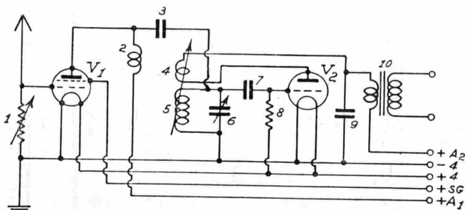
Fig. 3. — Circuito analogo al precedente ma semplificato. 1 = resistenza variabile da 50.000 ohm; 2 = bobina di « choke »; 4 = bobina di reazione; 5 = bobina a nido d'api; V_1 = valvola a placca schermata; V_2 = triodo normale.
