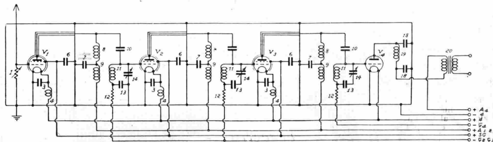
Fig. 5. — Circuito con tre stadi di amplificazione ad A.F. a valvole schermate.
