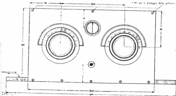
Vista anteriore del pannello
