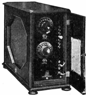
Apparecchio ricevente con diffusore completamente alimentato dalla corrente di illuminazione
