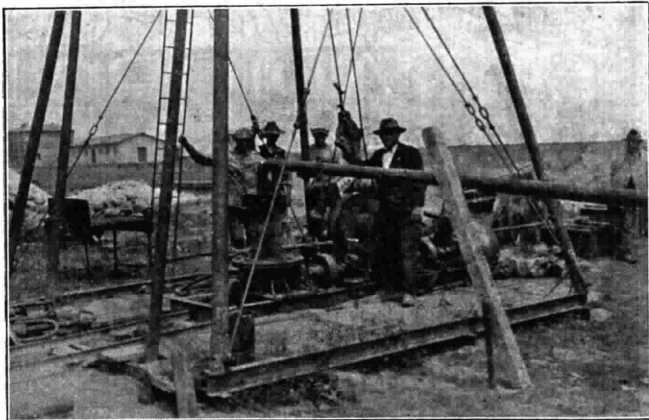
Fig. 3 - Perforazione del suolo per l'impianto di presa d'acqua (profondità m. 68)
