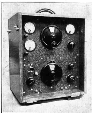
La Stazione radio portatile della ditta Allocchio Bacchini e C. di Milano di cui è dotata la spedizione Albertini
