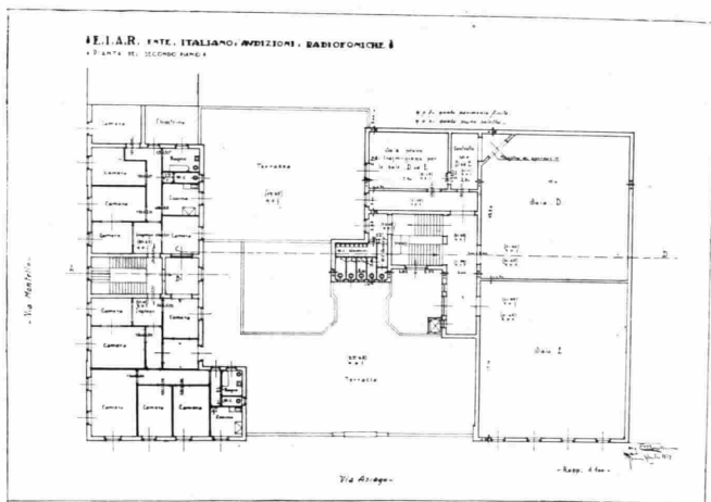
Pianta del secondo piano (quarto effettivo), col sesto e settimo auditorio.
