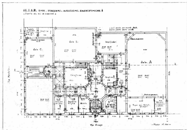
Pianta del piano rialzato (secondo effettivo), coi quattro auditori.
