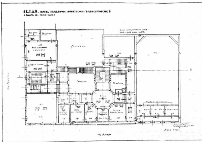
Pianta del primo piano (terzo effettivo), col quinto auditorio.
