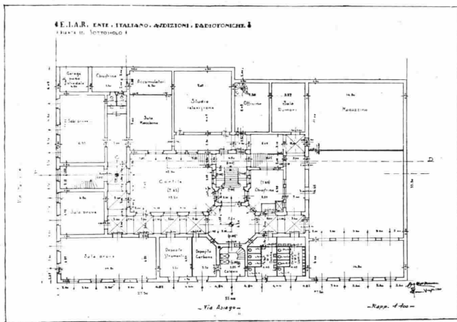
Pianta del semisottoterraneo (primo effettivo). Si notino le grandi sale previste per le prove degli elementi musico-lyrici, un grande salone d'aspetto e lo speciale studio per la televisione.
