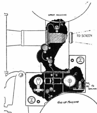
Principio della macchina per la proiezione dei film sonori sistema «Moviétone» e «Photophone» ed analoghi.
