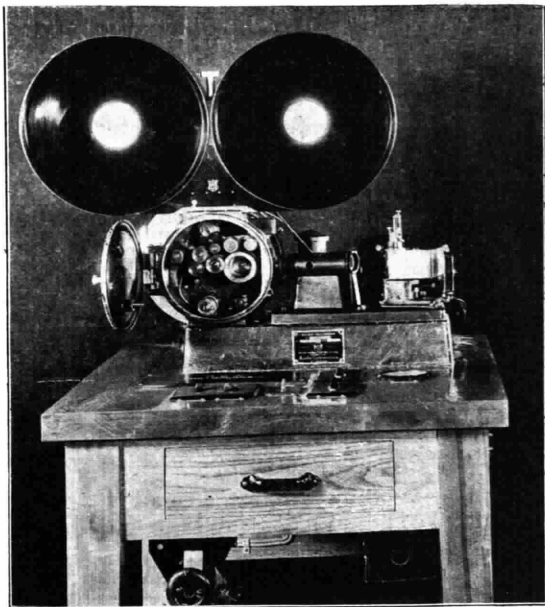
Dispositivo di registrazione dei suoni sulla pellicola - Sistema « Photophone ».
