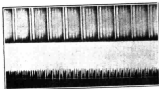
Tipi di registrazioni ottico-acustiche. Superiormente: sistema a densità variabile. Inferiormente: sistema ad area variabile.
