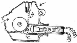
Principio di registrazione dei suoni, col sistema «Moviétone».
