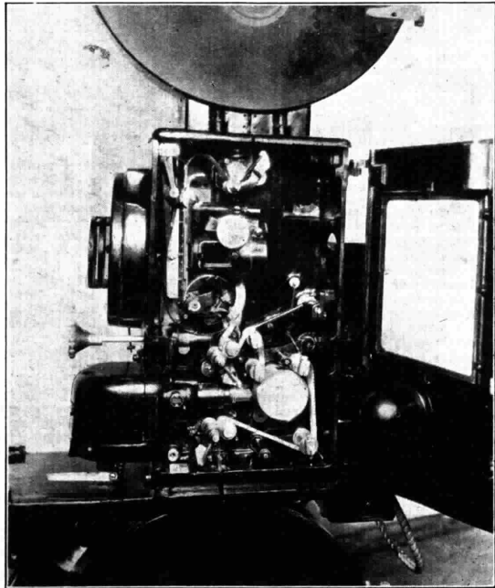
Proiettore Photophone. Dettaglio del sistema riproduttore a cella fotoelettrica.
