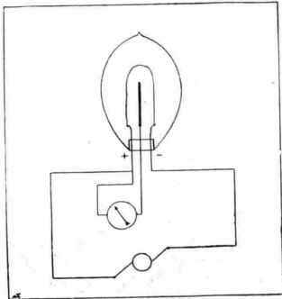
Fig. 4. — Circuito dimostrativo dell'effetto Edison
