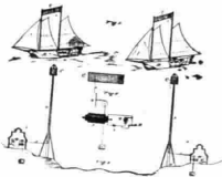
Fig. 3. — Apparecchio per la trasmissione di segnalazioni elettriche a distanza. (Dicembre 1891).
