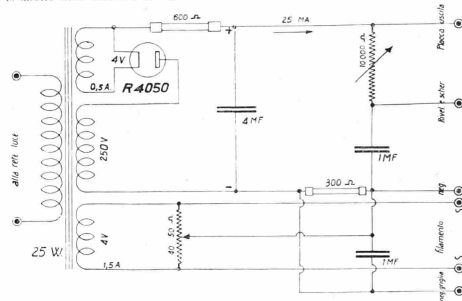
Fig. 1. Alimentatore totale per piccoli apparecchi.
