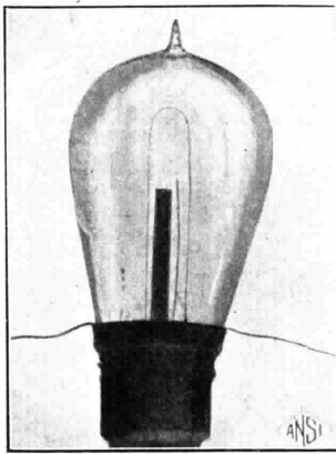
Fig. 6. — Una delle lampadine usate da Edison per lo studio dell'effetto Edison
