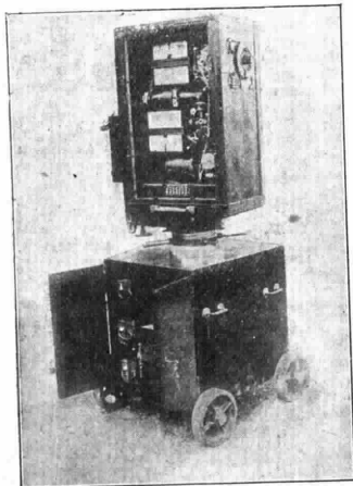
Dispositivo registratore dei suoni secondo il sistema Tri-Ergon
