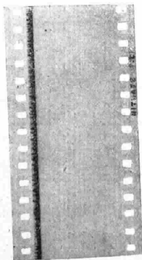
Registrazione fonica Photophone su pellicola separata
