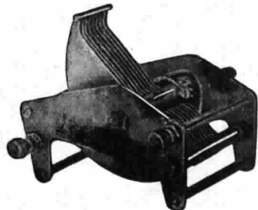
Tipo C. in ottone placche lat. nichelate su cuscinetti a sfera a variazione logaritmica.
