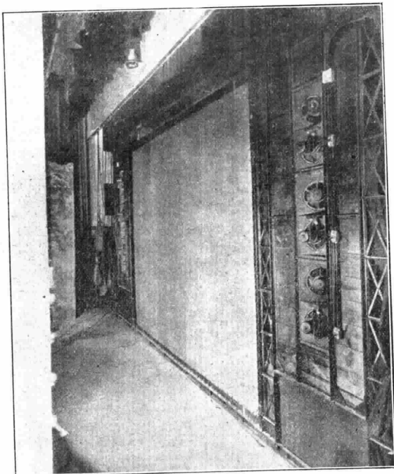
Installazione di otto altoparlanti elettrodinamici ai lati dello schermo di proiezione (vista dalla parte posteriore)
