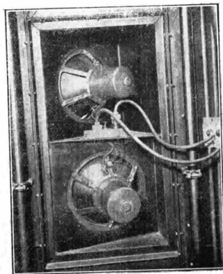
Altoparlanti elettrodinamici usati nell'impianto Photophone di riproduzione
