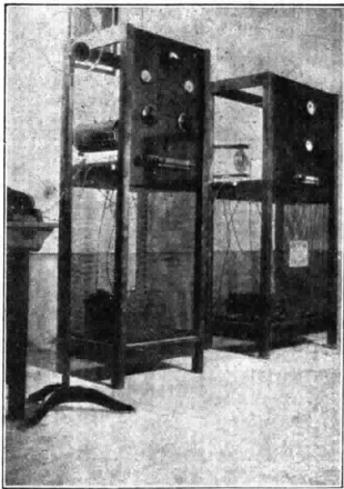
I pannelli della stazione RT e T S F della Legione « Leonessa »
