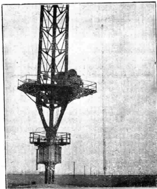
Torre della Stazione di Rugby per il servizio radiotelefonico con New York
