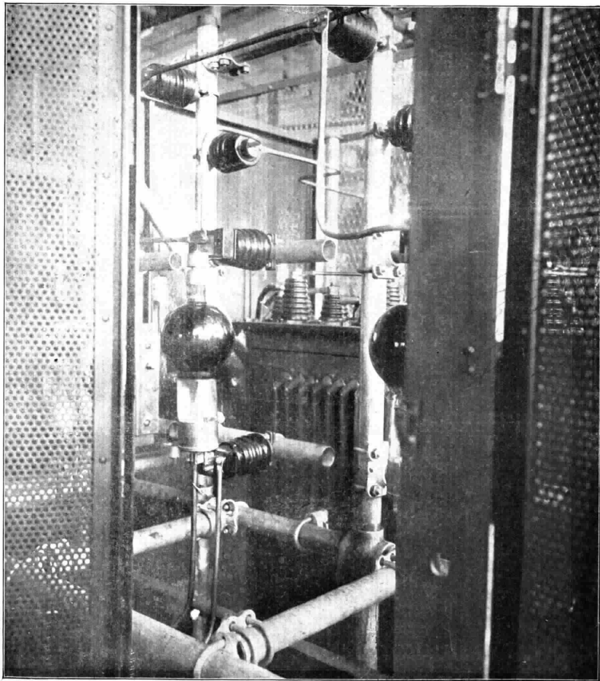
Rettificatore a vapore di mercurio (hot-cathode) della R.C.A. per la STAZIONE NAZIONALE DI ROMA DA 50 KW.
