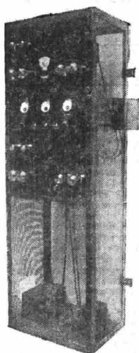
Doppio amplificatore «Fedi», per sale fino a 1200 posti. — Complesso amplificatore composto di doppio pannello, utilizzabile al totale o per metà quando si voglia disponibile una riserva. Le singole parti, fra le quali valvole, strumenti di misura e comandi, sono disposte su due distinti pannelli, affiancati da una robusta intelaiatura in ferro, nel fondo della quale trovano posto i trasformatori di riduzione della tensione della rete.
