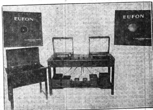
Tavolo di commento musicale dei films muti; accessorio indispensabile dell'impianto sincrono, che permette di avere sempre disponibile una buona orchestra radiofonica.
