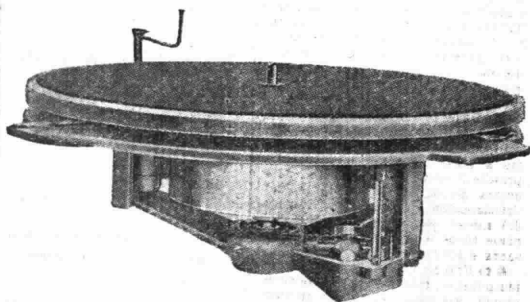
MOTORE AD INDUZIONE
