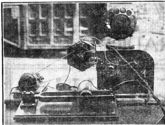
IL MICROFONO AD « ORECCHIO ELETTRICO »
