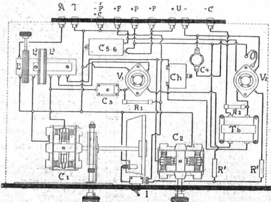
Piano costruttivo.
