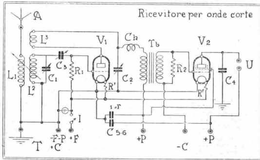
Schema elettrico.
