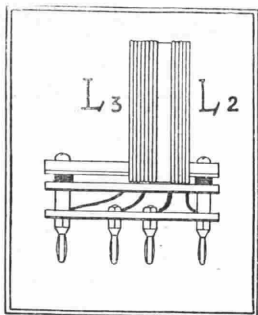
Dettaglio delle indutture (serie 2').
