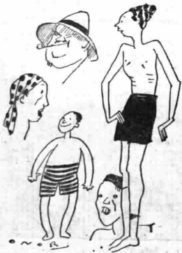
Tipi di « fumaroli ».
