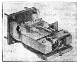
Figura 2 - Relais speciale ad alta frequenza
