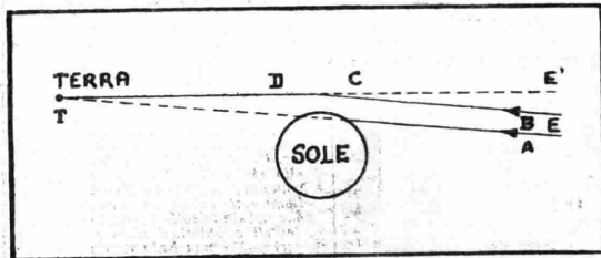
Il disegno indica la deviazione che un raggio luminoso BCDT proveniente da una stella lontana T o raggiungente la Terra T subisce in vicinanza del Sole. La parte iniziale BC e quella DT in realtà sono drittte ed un osservatore terrestre, ricevendo il raggio luminoso secondo DT, crede che la stella si trovi in questa direzione E' quindi in E', mentre senza la presenza del Sole egli riceverebbe tale raggio secondo la linea TA.
