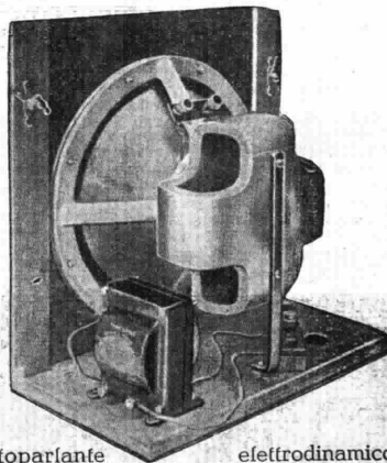
Altoparlante elettrodinamico con calamita permanente
