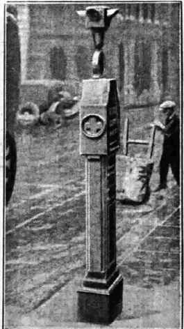
Un pilastro stradale di allarme per i poliziotti inglesi. Quando la centrale deve fare comunicazioni urgenti, il faro del pilastro si accende ed un campanello comincia a squillare
