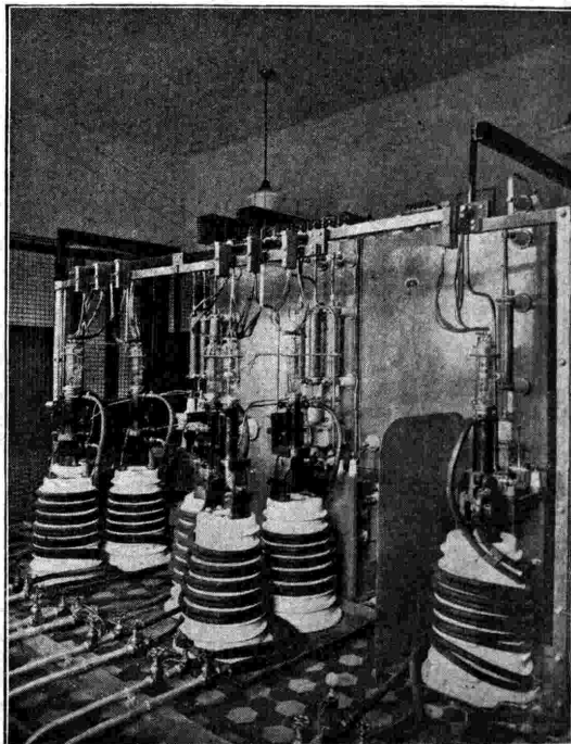
Trasmettitore di Firenze: lo stadio finale di potenza.
