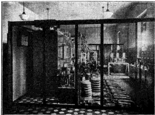
Il trasmettitore di Firenze. — Veduta laterale del complesso ad alta frequenza.
