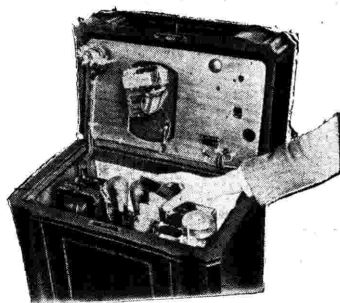
Il piano fonografico si solleva per accedere alle valvole.
