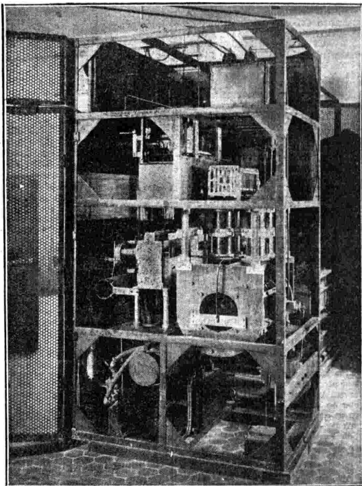
Vista posteriore pannello amplificatore intermedio (5 kW.).
