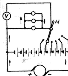
Circuito di carica
