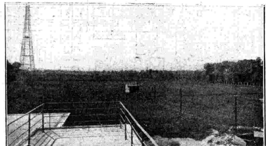
La linea di trasmissione ad alta frequenza e la cabina d'accordo d'antenna.
