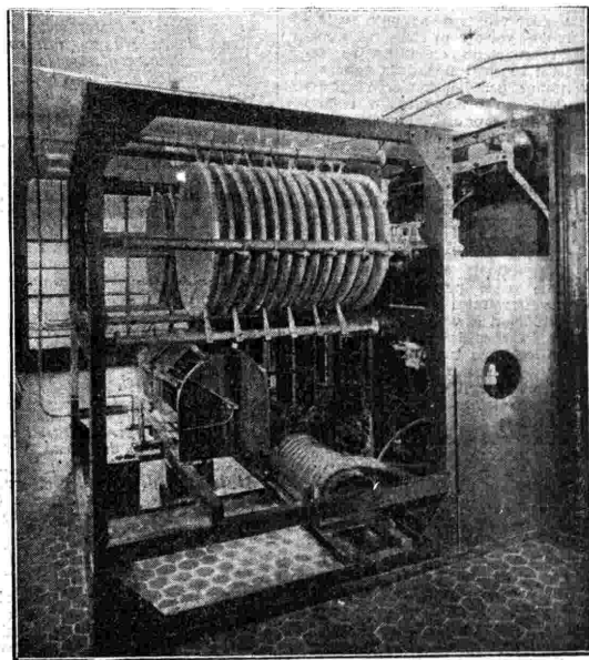
Vista posteriore pannello amplificatore di potenza (50 kW.).
