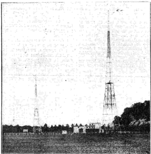
Vista generale del lato posteriore del trasmettitore di Siziano.
