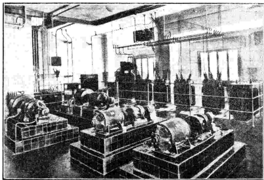
Dettaglio sala macchine.
