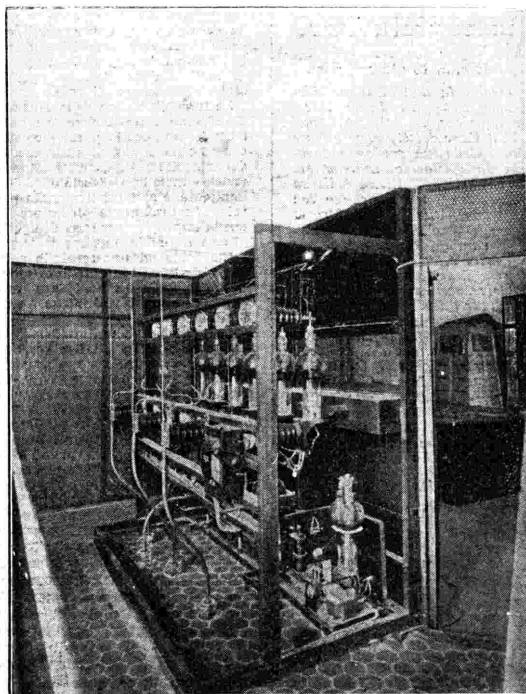
Vista posteriore pannello raddrizzatore di potenza (18.000 Volt - 10 Amp.).
