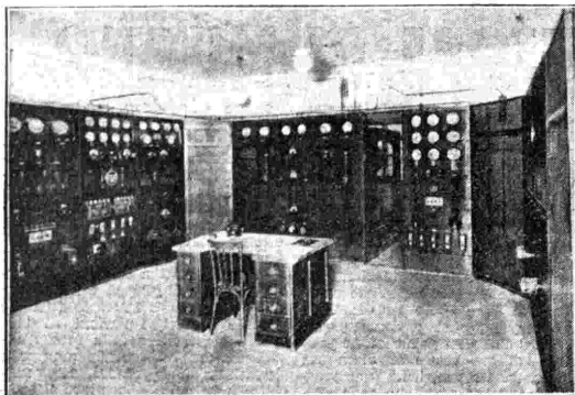
Sala pannelli alta frequenza.
