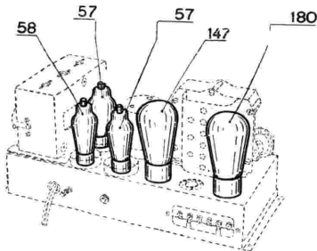
Fig. 3 - Lo «chassis».
