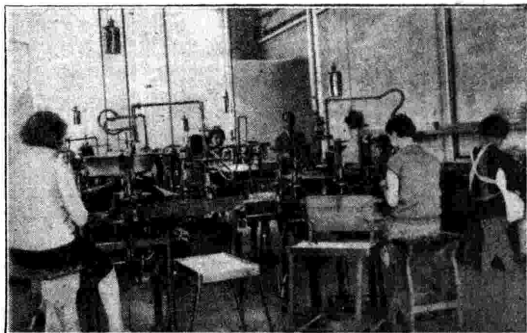
Macchine automatiche per la confezione dei supporti e per la chiusura delle valvole riceventi e trasmettenti.
