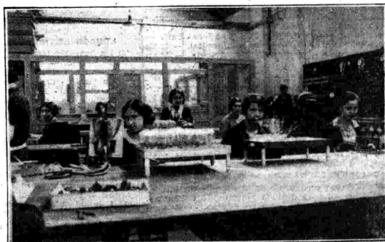
Salone per la zoccolatura e attivazione delle valvole.
