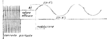
Fig. 1. - Modulazione a bassa frequenza di una corrente ad alta frequenza di valore efficace K con percentuale di modulazione K .
