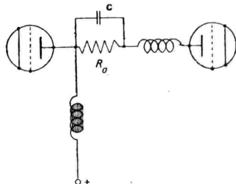
Fig. 3. - Variazione dello schema di Heising per modulare al 100%.
