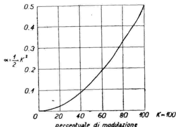
Fig. 2. - Valore relativo della potenza supplementare da fornire all'aereo per la formazione delle frequenze laterali in funzione del grado di modulazione.
