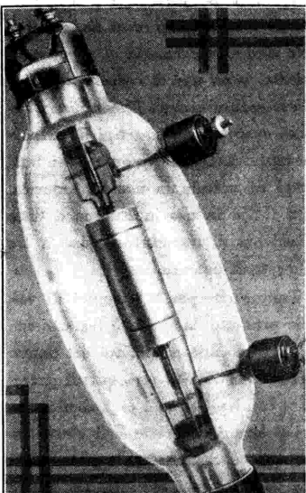
Valvola trasmittente: potenza dissipata un kilowatt.
