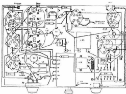
Fig. 2 - Schema costruttivo. Parte inferiore dello chassis.
