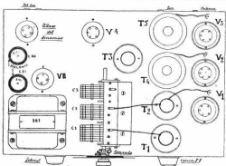
Fig. 2 - Schema costruttivo. Parte superiore dello chassis.
