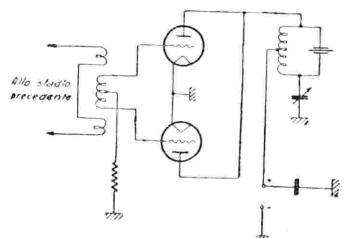
Schema di principio di duplicatore di frequenza.
