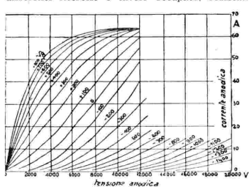
Caratteristiche statiche di un triodo da 100 kW.
