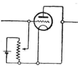
Oscillatore di Barkhausen e Kurz.
