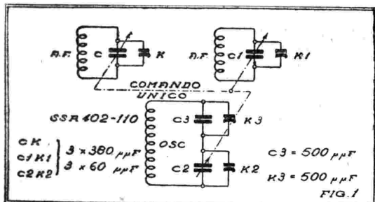
Il comando unico di una super eterodina con un condensatore triplo a tre elementi uguali.
