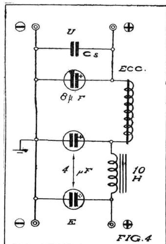
Esempio tipico di filtro provvisto di prefiltro e di condensatore supplementare.
