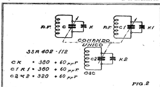
Il comando unico di una super eterodina mediante un condensatore speciale con settore per l'oscillatrice, sagomato.
